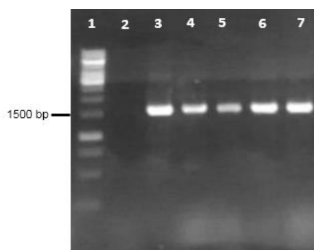
Hình 3. Kết quả PCR khuẩn lạc với cặp mồi đặc hiệu. 1: Thang DNA 1 kb; 2: Chứng âm; 3: Gene fliC ; 4-7: PCR khuẩn lạc với cặp mồi đặc hiệu
